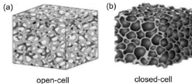
شكل (3) رسم توضيحي للخلايا المفتوحة (a) والمغلقة (b)
