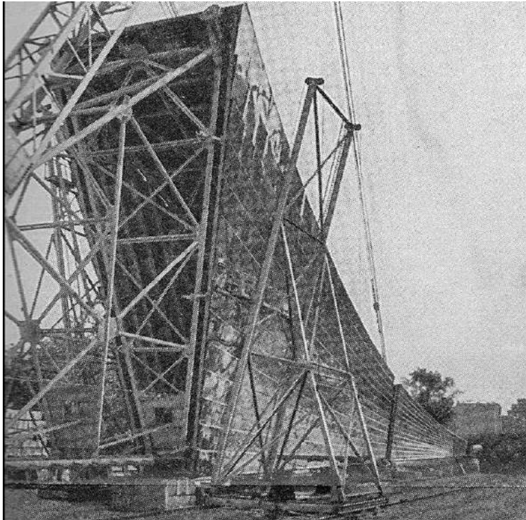
صورة رقم (٧) توضح تجميع الهيكل الشبكي الفولاذي الذي يزن ٢٥٠ طنًا يدويًا على الأرض وُرفِع بواسطة رافعات خاصة بجوار العمل
