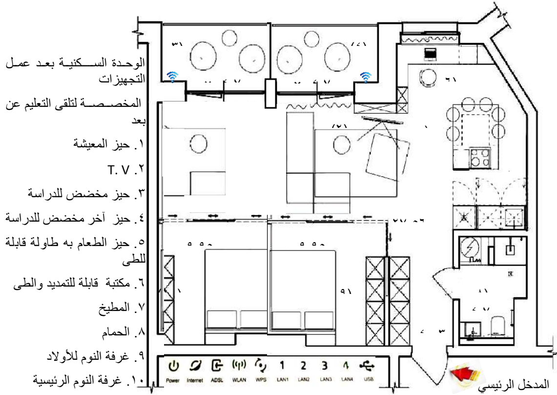
(شكل ٦) مسقط أفقي لدور السطح بوضوح توزيع الخدمات التكنولوجية على المبنى وتحويله إلى مبنى ذكي - مقياس رسم ١ : ٢٠٠
