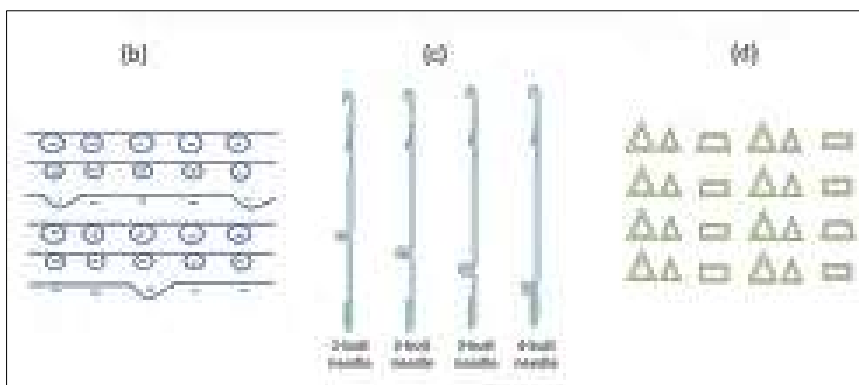
شكل (6، 7، 8): تركيب الغرزة والإبر وأنماط الكامات المستخدمة في إنتاج قماش الملون الحقيقي. (20)
