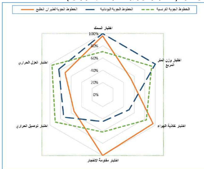
شكل (15): تحليل الأقمشة وتحديد أفضل ثلاث عينات ملائمة لطائرات الطائرات
