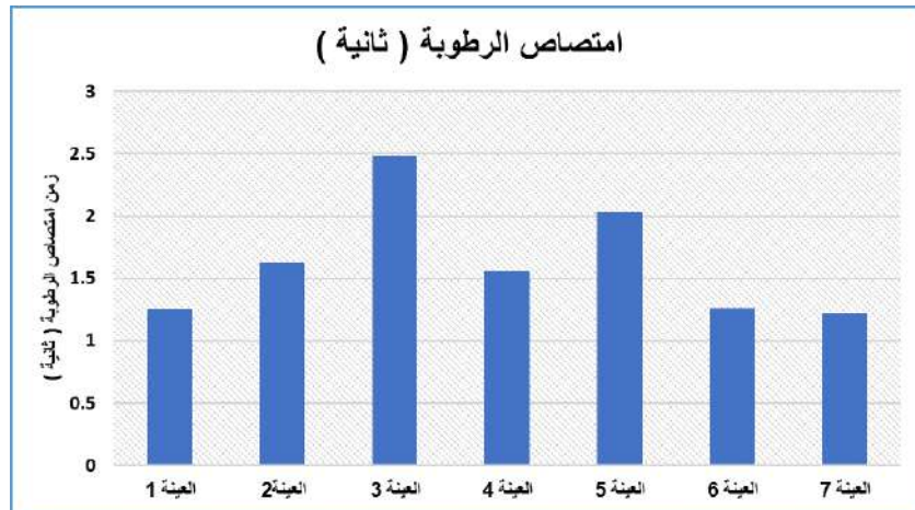
شكل (13): يوضح نتائج اختبار امتصاص الرطوبة (ثانية) للعينات المختلفة
