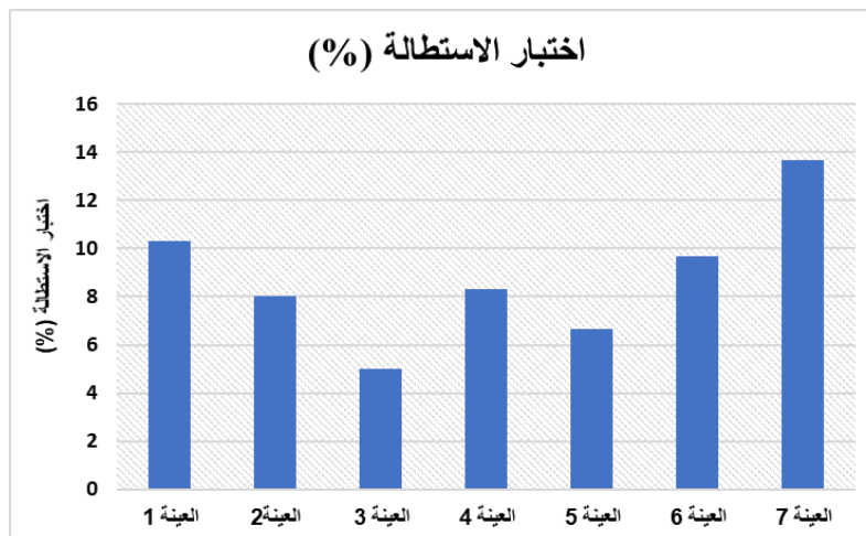
شكل (9): يوضح نتائج اختبار الاستطالة (%) للعينات المختلفة
