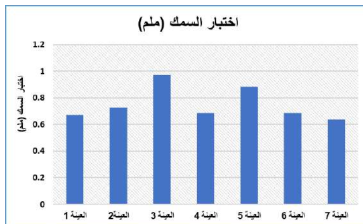
شكل (7): يوضح نتائج اختبار السمك (ملم) للعينات المختلفة
