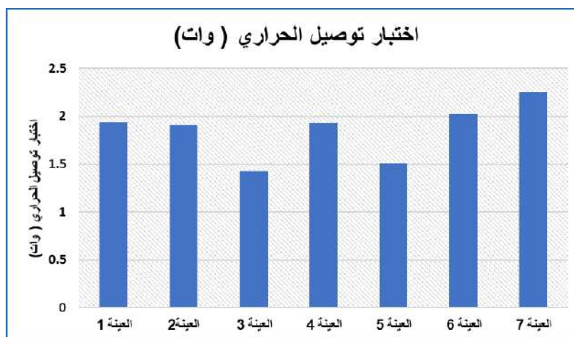
شكل (11): يوضح نتائج اختبار توصيل حراري (وات) للعينات المختلفة
