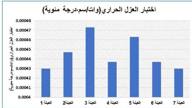
شكل (12): يوضح نتائج اختبار العزل الحراري (وات/سم 5 ) للعينات المختلفة
