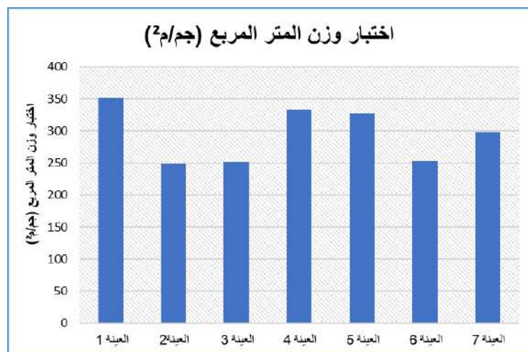
شكل (6): يوضح نتائج اختبار وزن المتر المربع (جم/م 2 ) للعينات المختلفة
