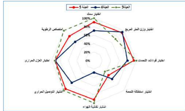
شكل (14): يوضح تحليل الأقمشة وتحديد أفضل ثلاث عينات مناسبة لاستخدامها في صناعة المعاطف
