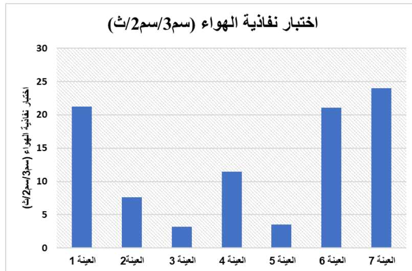
شكل (10): يوضح نتائج اختبار نفاذية الهواء (سم³/سم²/ث) للعينات المختلفة
