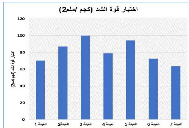
شكل (8): يوضح نتائج اختبار قوة الشد (كجم/ملم²) للعينات المختلفة
