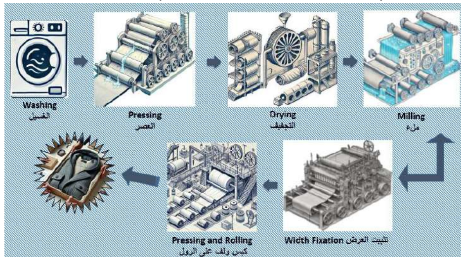
شكل (2) : يوضح مراحل عملية التجهيز التي تمر عليها المعاطف الشتوية شديدة البرودة
