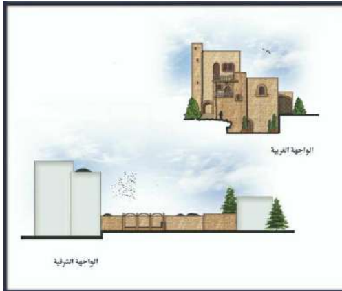
الواجهة الشرقية والغربية لمبنى النتشة 14
