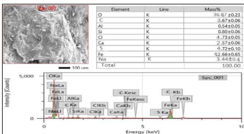
شكل رقم (١٥) يوضح تحليل ب EDX لعينة حديد شبائك قلعة قايتباي ٢٠٢٣.
