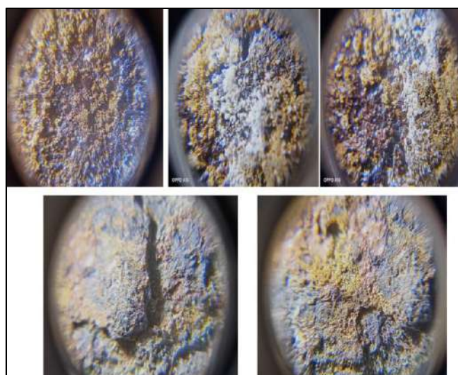
شكل رقم (٦) يوضح طبقات التآكل على سطح الحديد الاثري
