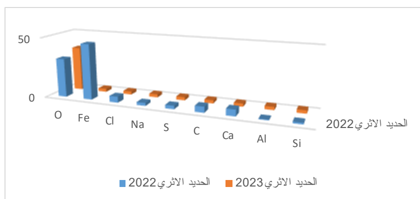
شكل رقم (١٧) يوضح مقارنة التحليل بـ EDX عينات حديد شبائيك قلعة قايتباي.
