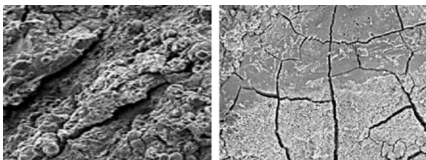
شكل رقم (١٦) يوضح الشقوق والكسور في طبقات التآكل وعدم استواء طبقة التآكل لعينة الحديد الأثري ٢٠٢٣
