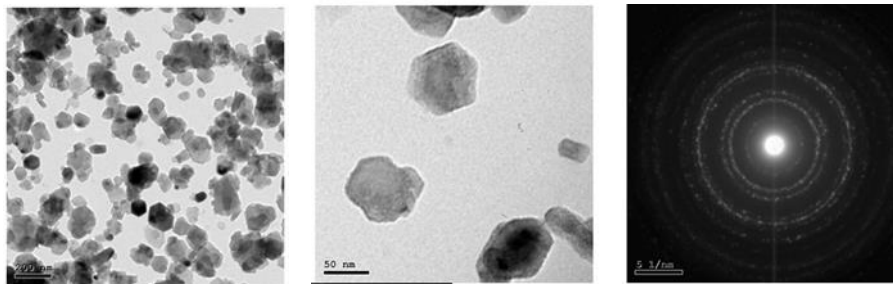
صورة (١١) عينة نانو هيدروكسيد الكالسيوم تحت الميكروسكوب الاليكتروني النافذ TEM بتكبير X3000, X30000, X4000
