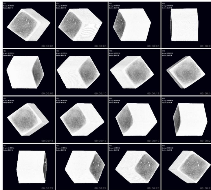
صورة (١٥) ثلاثية الابعاد DCT بتقنية التصوير المقطعي للعينة بعد التقوية وتوضيح الانتشار المتجانس لنانو هيدروكسيد الكالسيوم علي السطح الخارجي للالباستر المصري ويتضح ذلك من خلال الزوايا المتعددة والمختلفة لعينات الالباستر المصري
