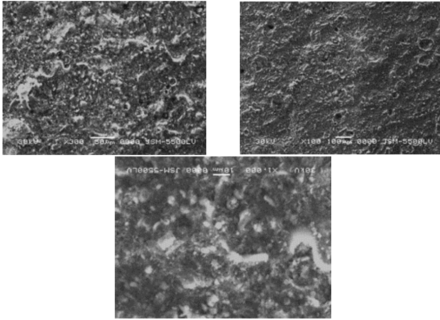
صور (١٢، ١٣، ١٤) من خلال الفحص بالميكروسكوب الاليكتروني الماسح حقق نانو هيدروكسيد الكالسيوم نجاحا وثباتا ملحوظا في تقوية الالباستر من حيث القدرة علي الربط المتجانس لنانو هيدروكسيد الكالسيوم داخل المسام.
