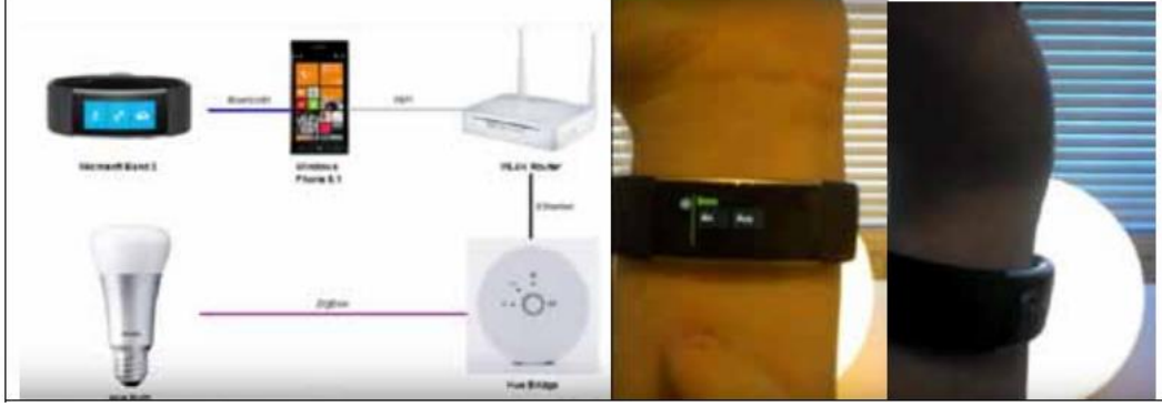
صورة (١٣) يوضح كيفية الربط بين الأجهزة القابلة للارتداء مثل Microsoft Band و Apple watch والتحكم بالاضاءة عن طريق منتجات شركة فيليبس Phillips Hue ويظهر في الشكل التحكم في الاضاءة عن طريق حركة الرسغ وذلك يتم من خلال قراءة حركة المجسمات الداخلية للأجهزة الذكية وربطها بالوحدة المضاءة.
