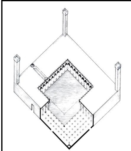
الشكل رقم (2): منظور للمسجد النبوي عقب عمارة (الوليد بن عبد الملك)، نقلاً عن: (Hillenbrand).
