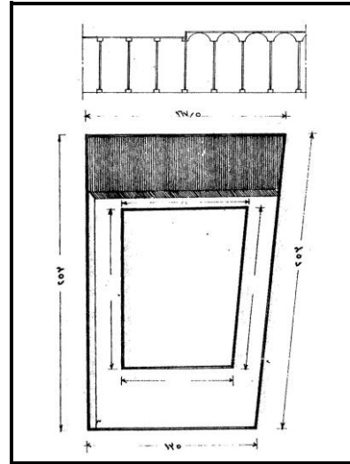
الشكل رقم (5): مسقط للمسجد النبوي، يوضح الجزء المرتفع من سقف المقدم بعد إضافة (الناصر محمد) بلاطني مقدم المسجد، نقلاً عن: (الشهري).
