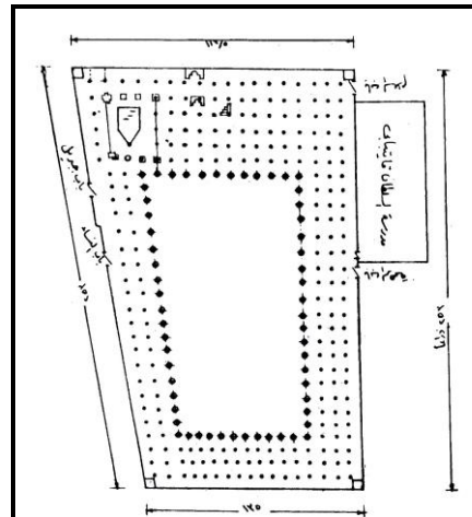
الشكل رقم (7): مسقط للمسجد النبوي، عقب عمارة (قائتباي) الثانية، نقلاً عن: (الشهري).
