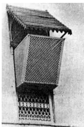
(صورة 10) : تبريد تيار الهواء المار عبر جرار المياه عن طريق عمليات التبريد التبخيري ووظيفة داخلية للتحكم في حركة الهواء والجزء العلوى من المشربية يسمح بخروج الهواء الساخن -
