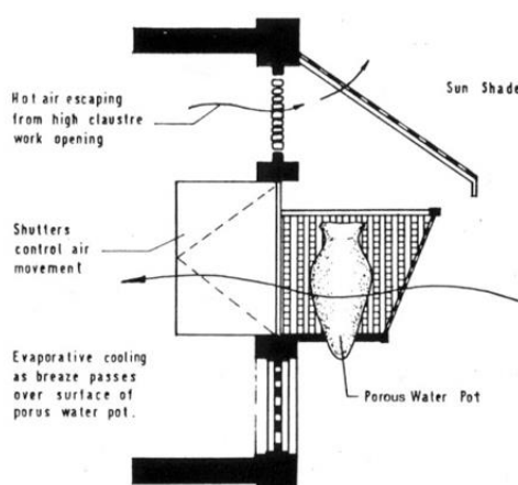
(صورة 10) : تبريد تيار الهواء المار عبر جرار المياه عن طريق عمليات التبريد التبخيري ووظيفة داخلية للتحكم في حركة الهواء والجزء العلوى من المشربية يسمح بخروج الهواء الساخن -
