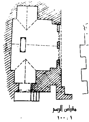
شكل (3) مدرسة الخيرية حسن - مسقط أفقي - - نقلاً عن :
