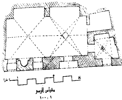
شكل (4) المدرسة العجمية - مسقط أفقي - نقلاً عن :
