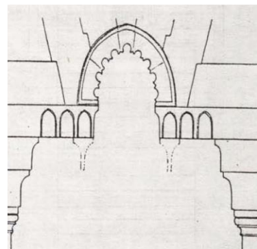
شكل (5) العقد المفصص لطاقية مدخل جامع بشتاك - نقلاً عن : دللي: العمارة العربية، لوحة 52
