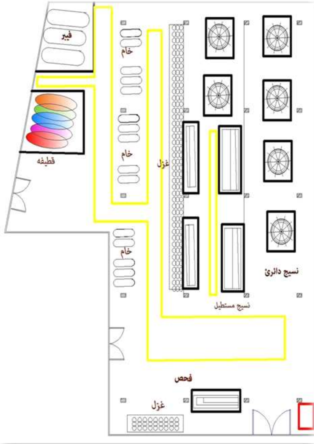
شكل (7) رسم كروكي للمسقط الافقي للفراغ بعد تعديل مسارات الحركة وأماكن المعدات والأثاث
