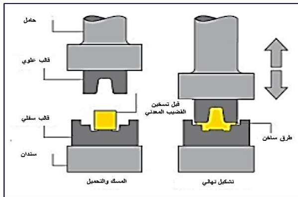
شكل رقم (٦) انسياب المعدن أثناء التشكيل بقوالب الحدادة المغلفة www.mechanicalengineeringblog.com
